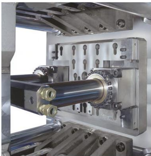
Piastra bloccaggio automatico estrattori. Plate to lock ejection automatically.
